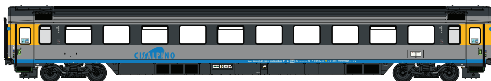
EC Apm
