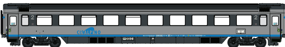
EC Bpm
